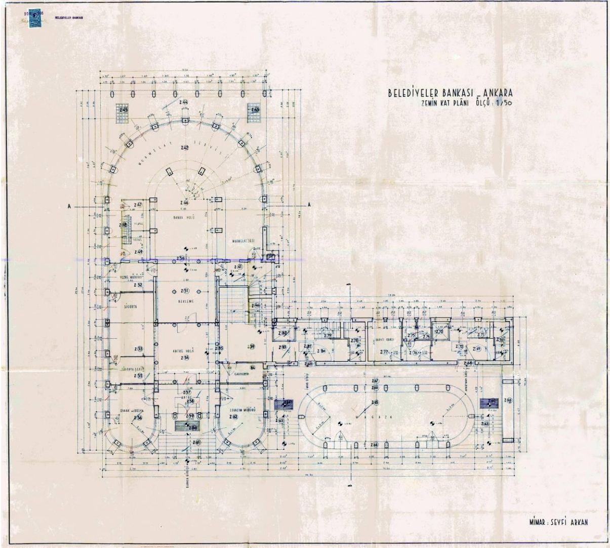
Şekil 1. Zemin kat planı
