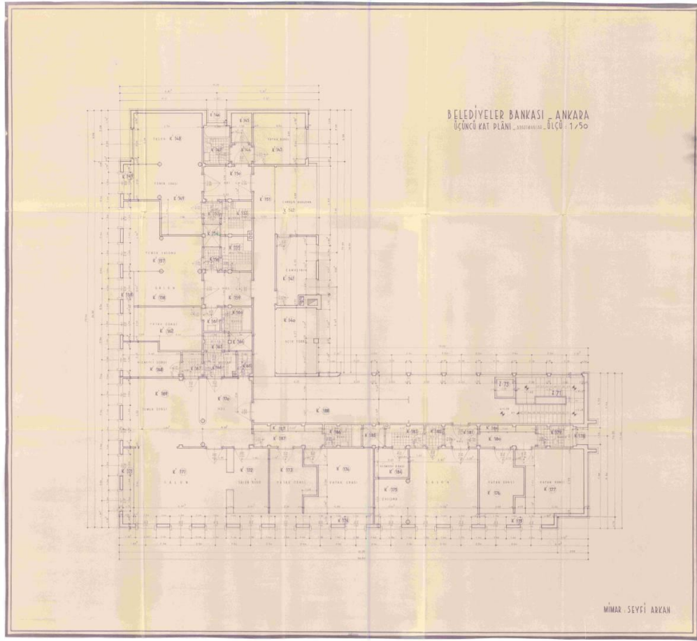
Şekil 4. Üçüncü kat planı
