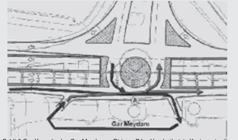
Şekil-3 Gar Kavşağından Gar Meydanına Giriş ve Çıkış Hareketlerinin Kesişmesi
