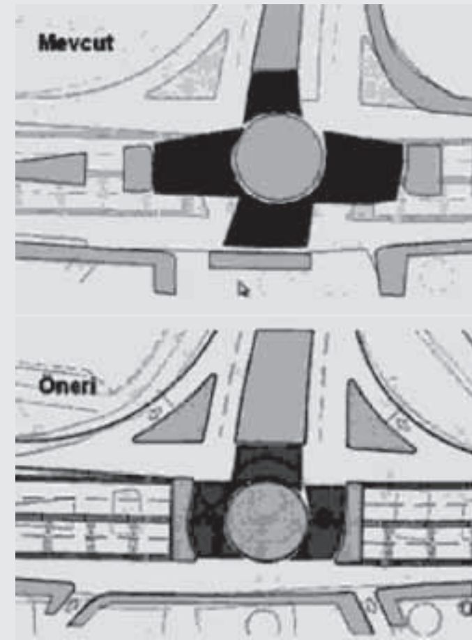
Şekil-2 Gar Kavşağı Sol Dönüş Depolama Alanlarının Küçülmesi
