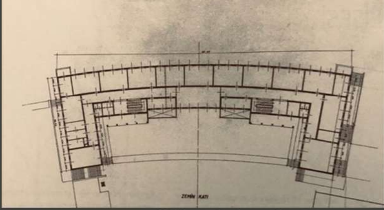
ANKARA KIZ LİSESİ PROJESİ / M. 1:200
