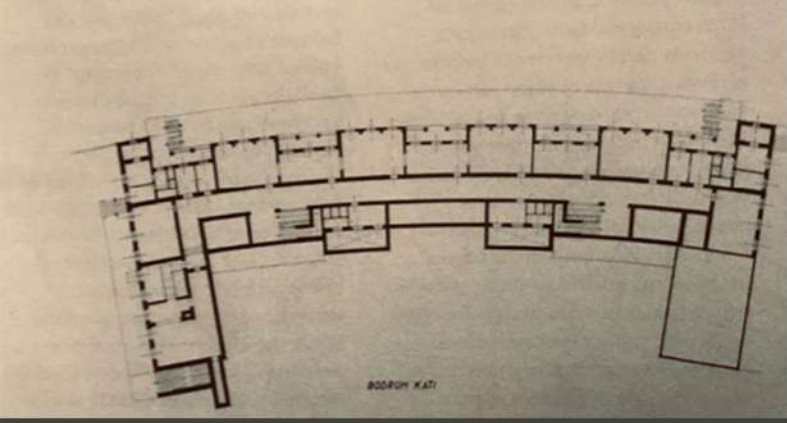
ANKARA KIZ LİSESİ PROJESİ / M. 1:200
